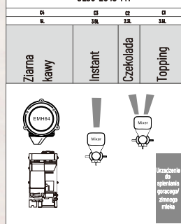
Układ modelu JL35-ES4C-FM
