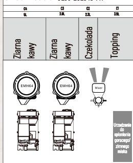
Układ modelu JL35-ESLC4C-FM
