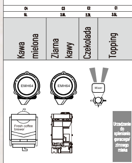
Układ modelu JL35-ESBTC4C-FM
